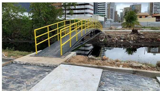
Construção de passarela para pedestres - Jardins
